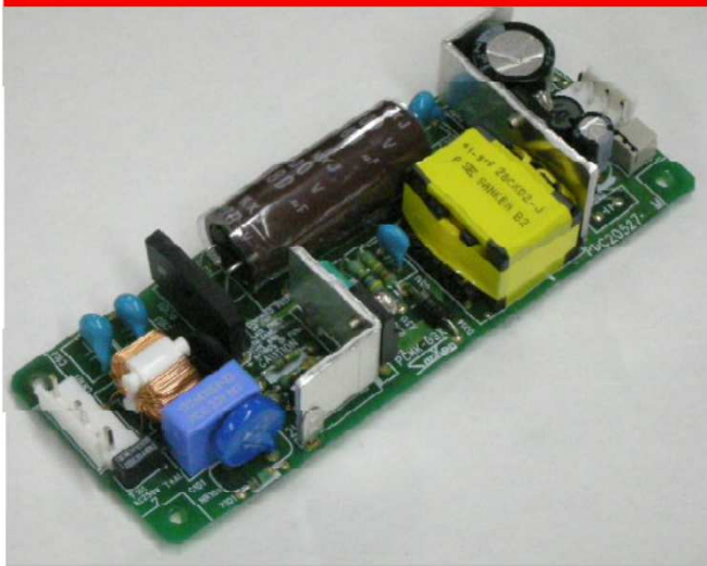
50W品 (SWF050P-24)
